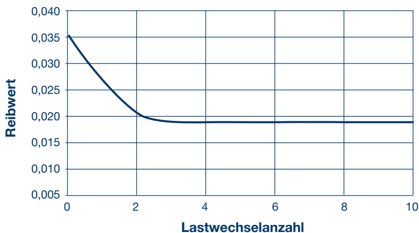
Bild 4: Reibwerte
