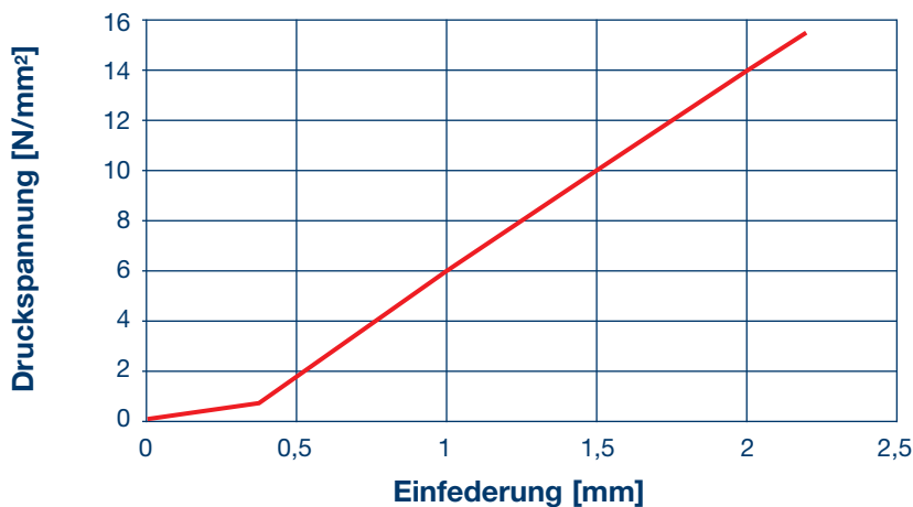
Bild 5: Einfederung \Delta t (näherungsweise)
