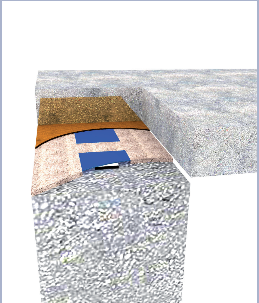
Bild 3: Einbau Civalit®-Streifengleitlager; Prinzipdarstellung
