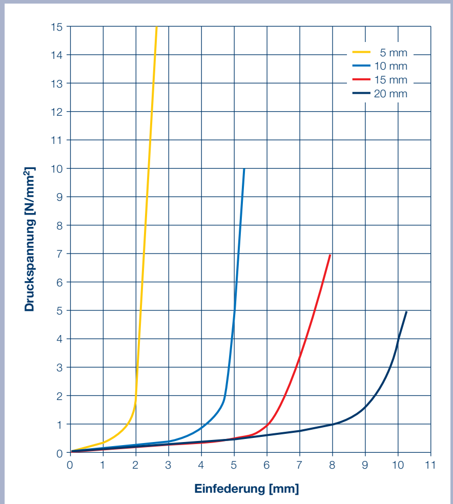
Bild 9: Lagereinfederung, Orientierungsdiagramm
