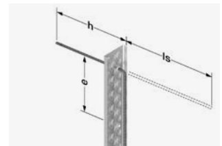
FERBOX® E03
