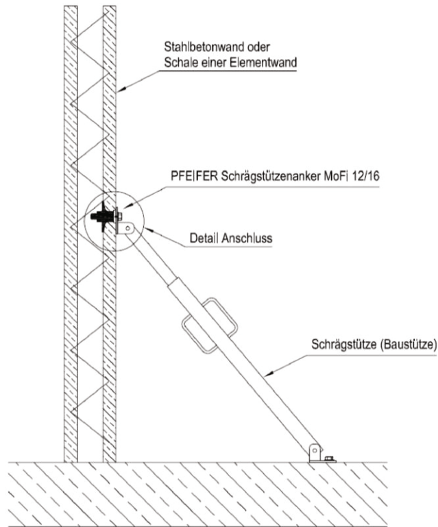
Bild 1: Beispiel einer Anwendung für h = h_{\min}
