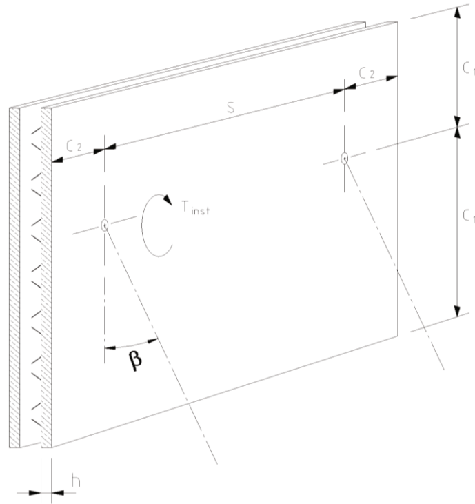
Bild 7: Mindestabstände, Neigungswinkel \beta der Stütze
