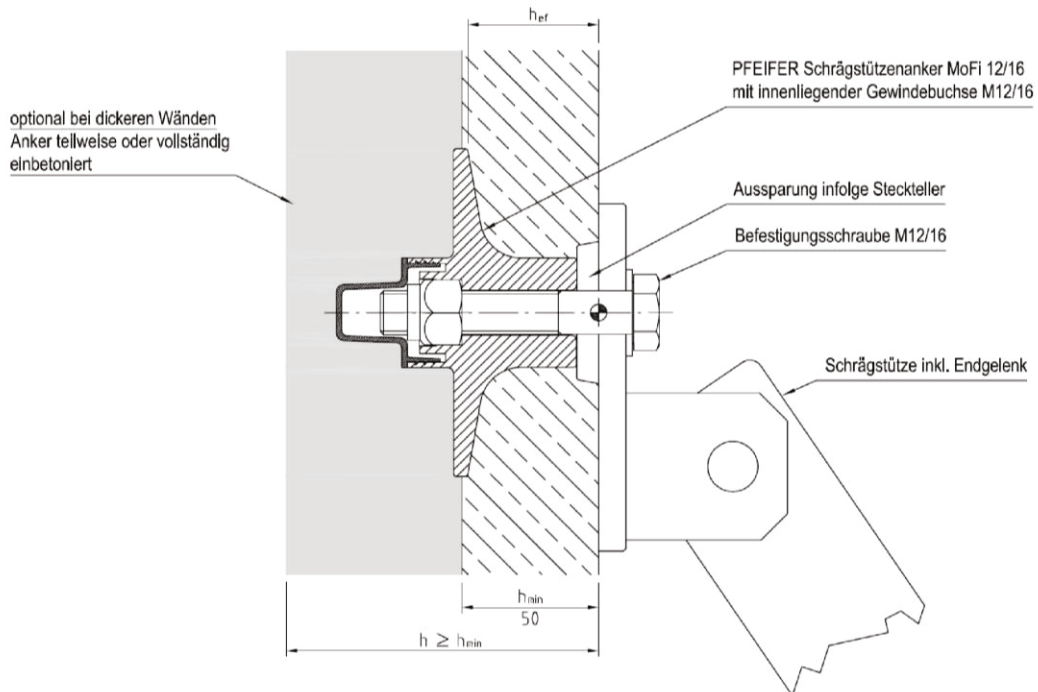
Bild 2: Detail Anschluss mit h = h_{\min} und h > h_{\min} (grau hinterlegt)
