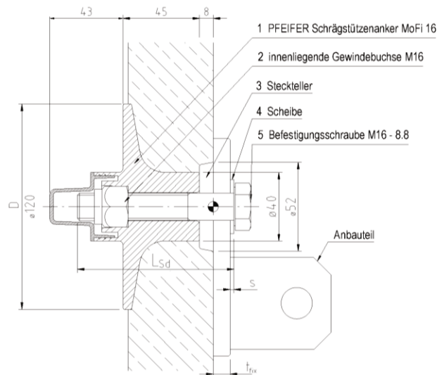
Bild 4: Bezeichnungen, Abmessungen MoFi 16
