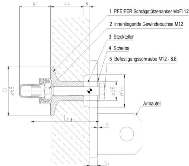
Bild 3: Bezeichnungen, Abmessungen MoFi 12
