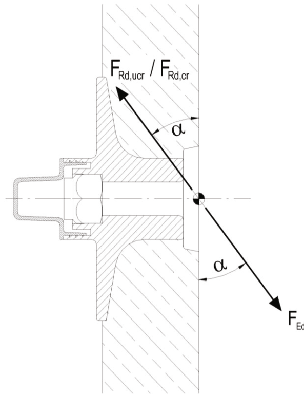
Bild 8: Definition des Widerstands mit Neigungswinkel \alpha des Widerstandes
