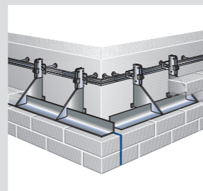
Vnější rohy s dilatačními spárami nebo bez nich
