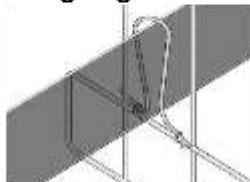
Omegabügel
