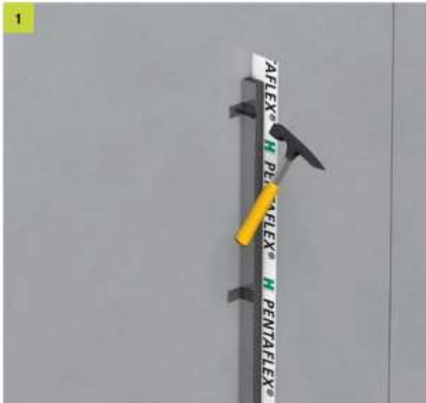
1 Das PENTAFLEX® Modul an den Nagellaschen an die Schalung nageln
