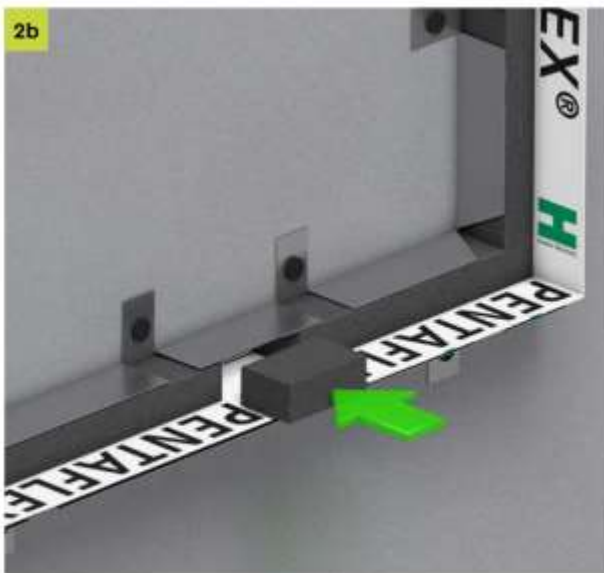
2b Leerräume mit EPP-Stopfen auffüllen
