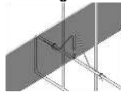
Klemmbügel
