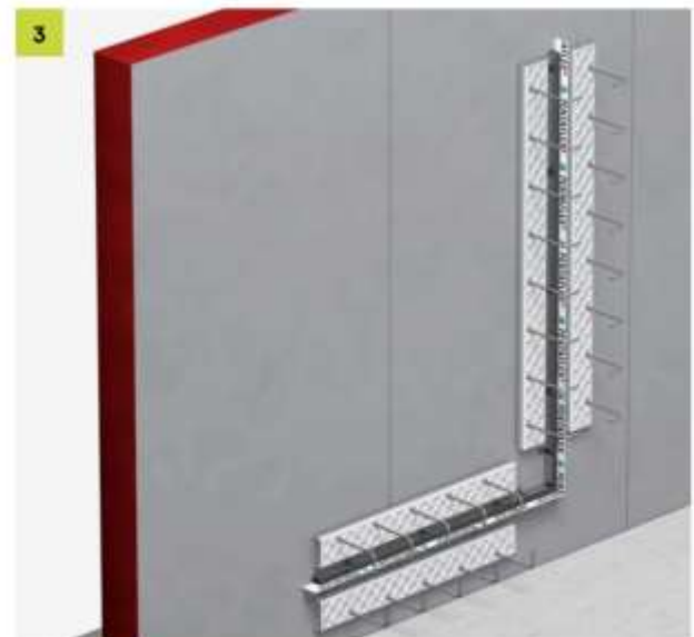
3 Neben das PENTAFLEX® Modul je zwei einreihige FERBOX® Rückbiegeanschlüsse an die Schalung annageln
