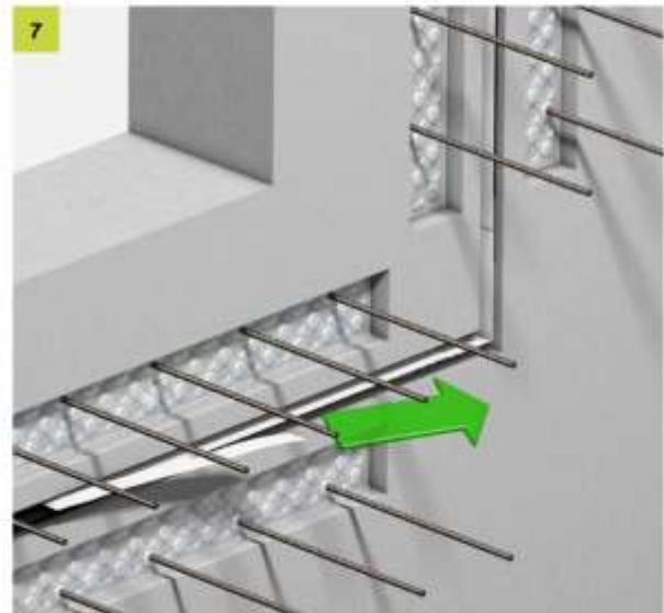
Die zweite Hälfte der Schutzfolie vom PENTAFLEX® Fugenblech abziehen. Anschließend den zweiten Betonierabschnitt schalen und betonieren
