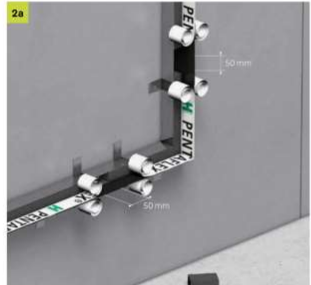
2a Verbinden des Eckmoduls mit zwei PENTAFLEX® Modulen:
