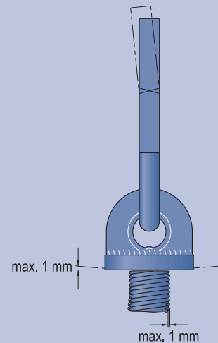
Bild 4: Ablegereife bei Verformungen
