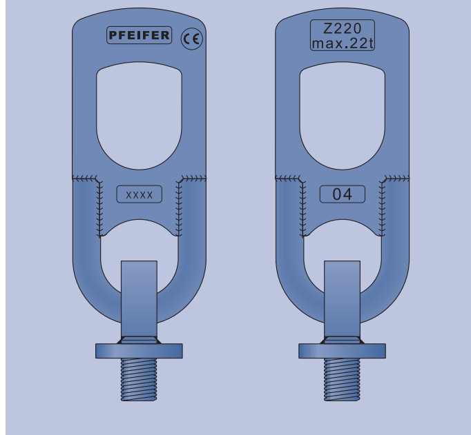
Bild 1: Kennzeichnung
