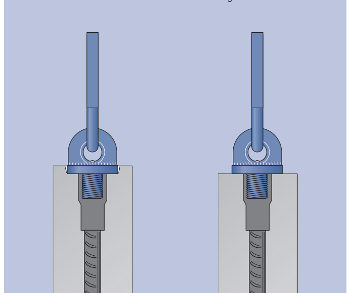
Bild 3: Passung des Superaufhängers...
