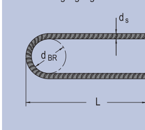
Bild 5: Zusatzbewehrung „Schrägzug in Plattenebene“
