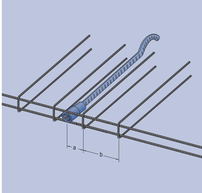
Bild 1: Mindestrundstahlbewehrung „zentrischer Zug“
