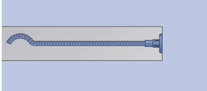
Bild 5: Sauberer Abschluß mit dem Verschlusssteller
