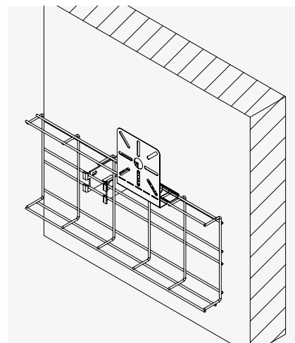
Montage der Montageplatte MP-G 90° zur Befestigung von Abzweigkästen an einer vertikal ausgerichteten U-förmigen Gitterbahn, hergestellt mit dem Gitterbahnverbinderset GV 30.
