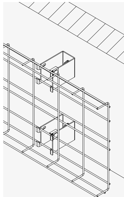
Horizontale Wandmontage einer vertikal ausgerichteten U-förmigen Gitterbahn, hergestellt mit dem Distanzbügel für Gitterbahnrastermaß 50 mm GBH 50.
