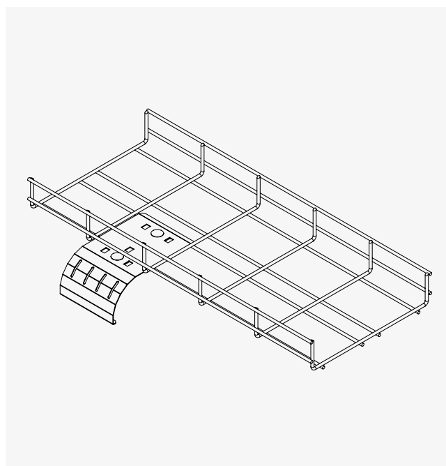
Montage des Abgangsblechs GKAB an einer U-förmigen Gitterbahn.
